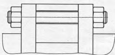
a) 单法兰
